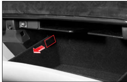
2. 글로브 박스 좌측 홀더 부분을 화살표 방향으로 당긴 후 돌려서 탈거하십시오.
