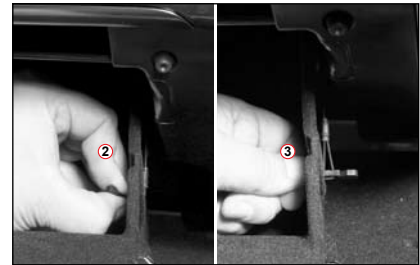
3. 글로브 박스 우측 부분의 고정 레버를 ②와 같이 들어올린 상태에서 ③과 같이 기울여 와이어링 연결 홀로 빼내십시오
