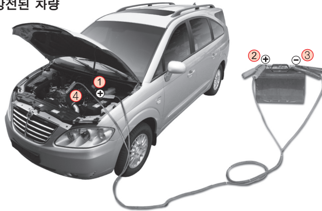
방전된 차량
